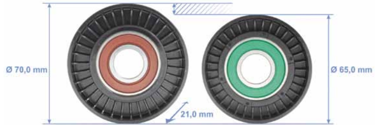
Şekil 2: Benzinli motora sahip araçlar için 532 0404 30 saptırma kasnağı (sol) ve dizel motora sahip araçlar için 532 0406 30 saptırma kasnağı (sağ)
